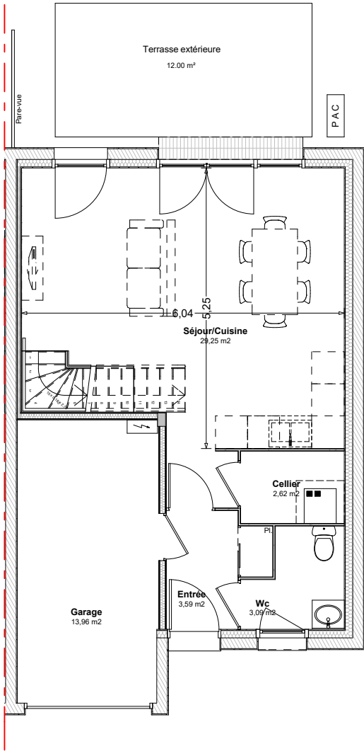
Rez-de-Chaussée
